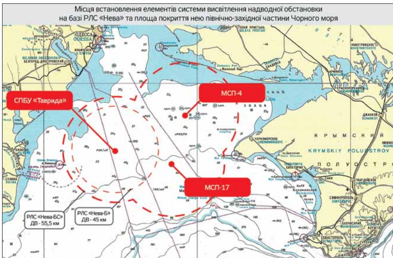
Рис. 2. Місця встановлення елементів системи висвітлення надводної обстановки на базі РЛС «Нева» та площа покриття нею північно-західної частини Чорного моря
