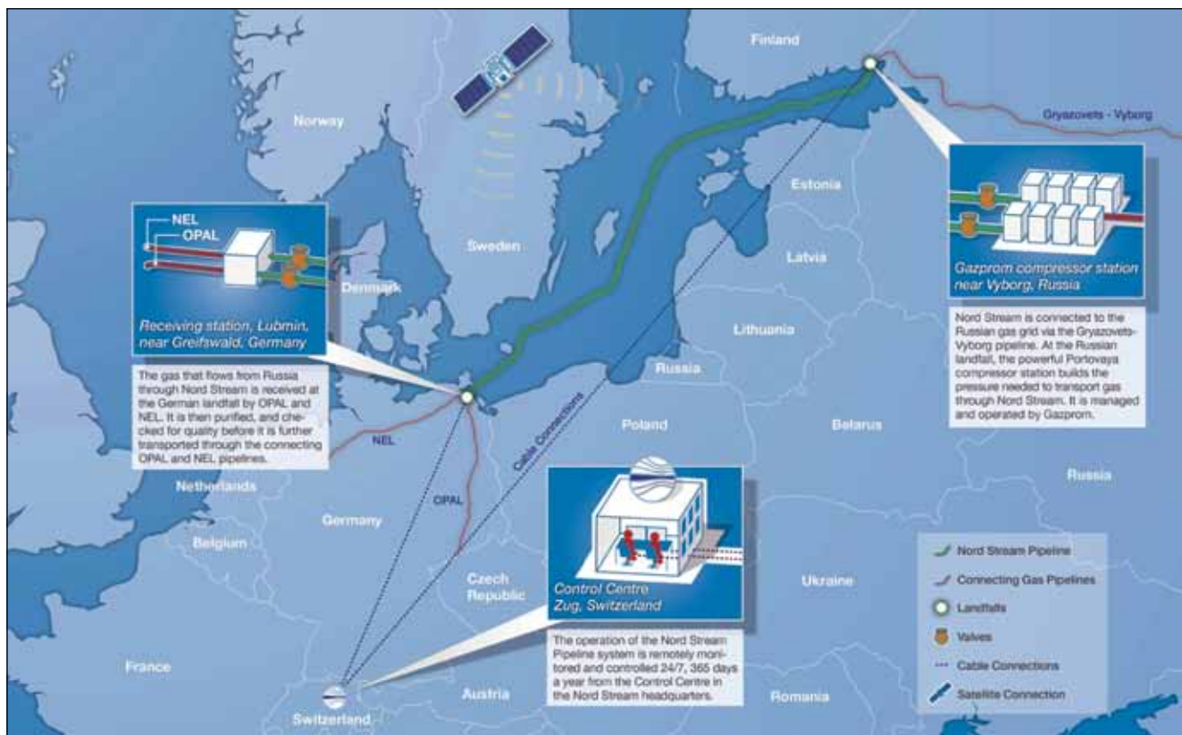
Рис. 4. Загальна схема управління трансбалтійською газотранспортною системою з офісним розміщенням Головного центру управління в Швейцарії, оснащеного оптоволоконним та супутниковим зв'язком. https://www.nord-stream.com/press-info/images/nord-stream-operation-facilities-3244/?q=&category=115&year=all&page=9&per_page=12
